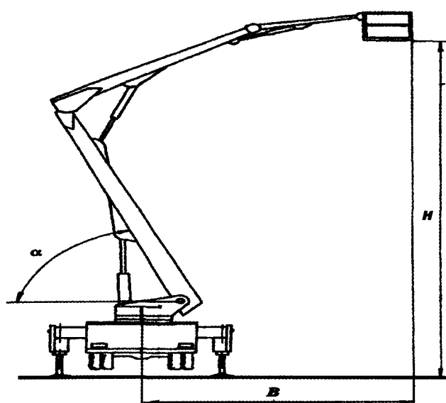
Рис. 2.2. Основные характеристики АПК: Н - рабочая высота; В - вылет; \alpha - угол подъема стрелы
