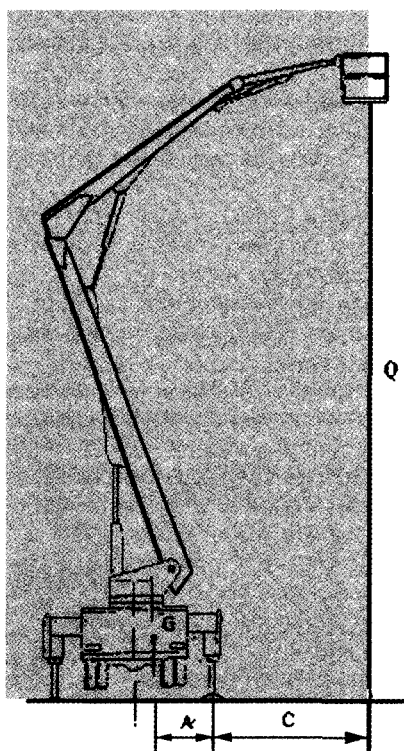
Характеристики для определения грузовой статической устойчивости пожарных АЛ (АПК)
