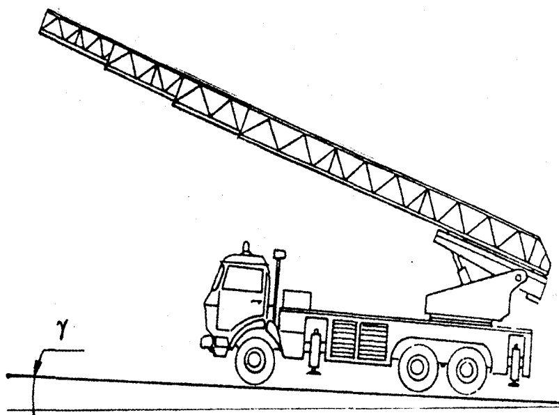
Продольный угол наклона АЛ: Y ~ продольный угол наклона
