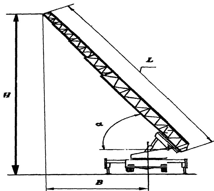
Рис. 2.1. Основные характеристики АЛ: Н - рабочая высота; В - вылет; L - длина лестницы; \alpha - угол подъема стрелы
